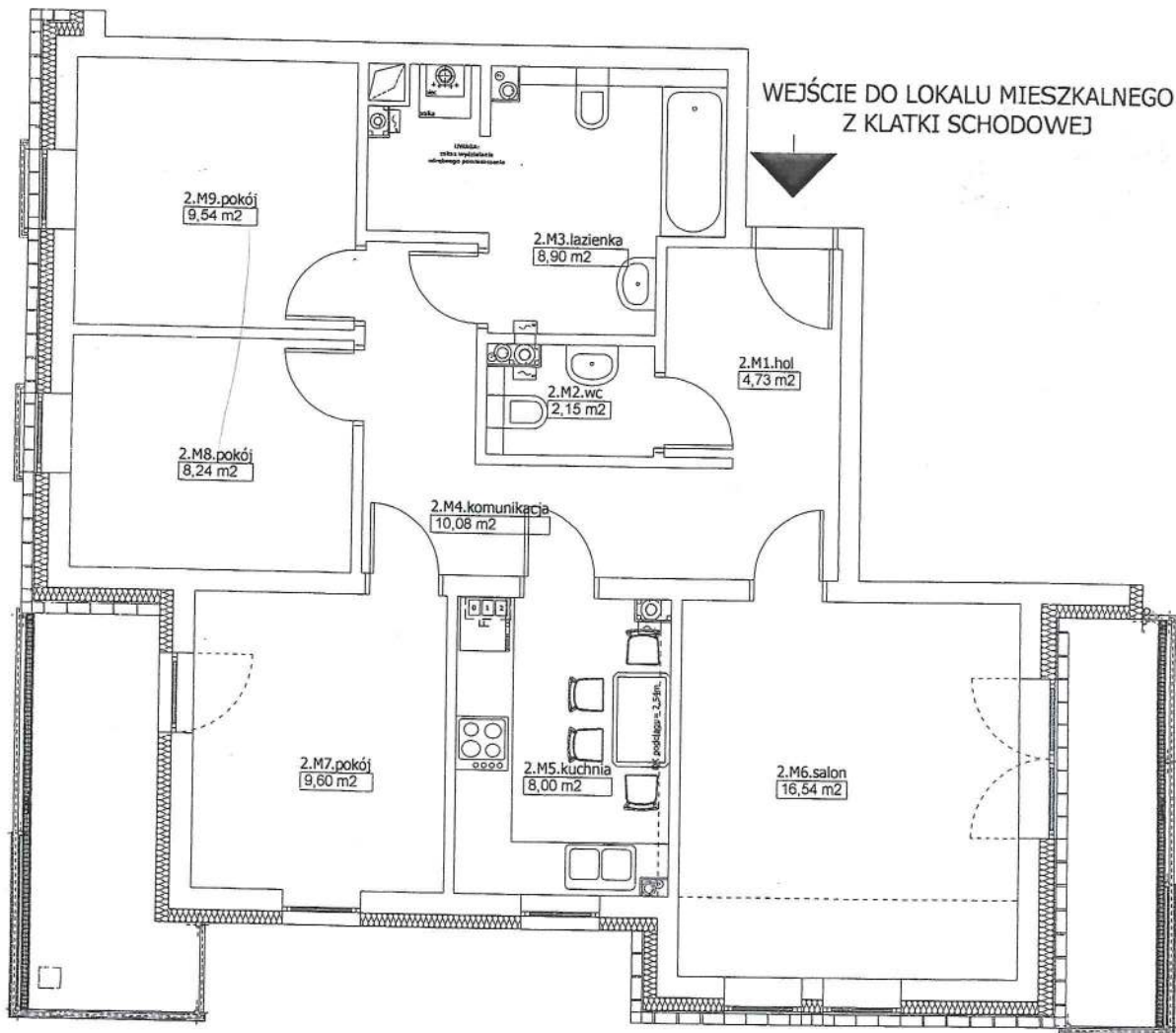
schemat rzutu mieszkania brak skali
